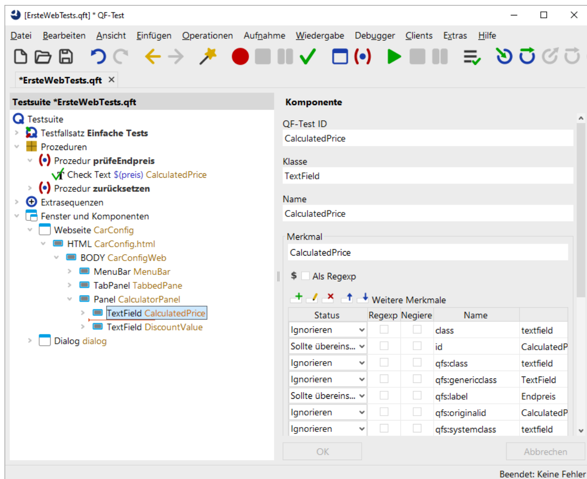
Abbildung 13.4: Komponentenbaum
