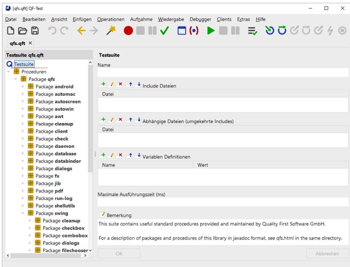
Abbildung 7.1: Die Standardbibliothek
