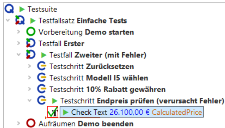
Abbildung 5.14: Korrigierter Check-Knoten
