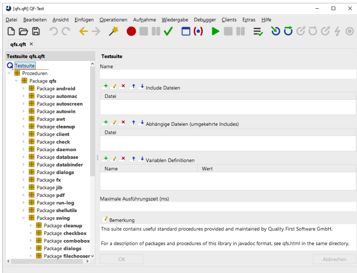
Abbildung 16.1: Die Standardbibliothek
