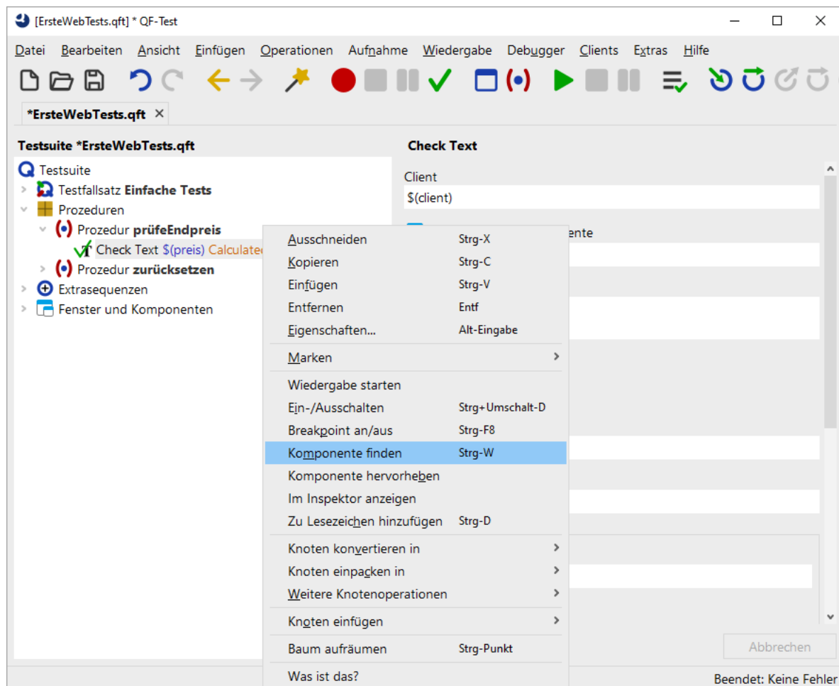
Abbildung 13.3: Komponente finden
