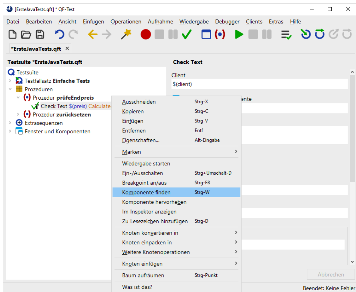
Abbildung 4.2: Komponente finden
